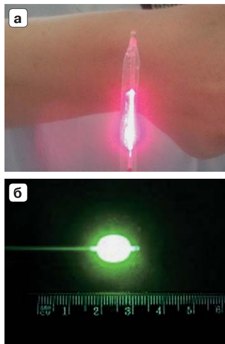
Рис. 6. Оптоволоконная система доставки лазерного излучения: а — световод с цилиндрическим рассеивателем; б — световод с баллонным рассеивателем.
