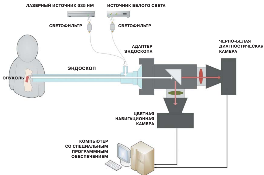
Рис. 2. Видеофлуоресцентный модуль.
